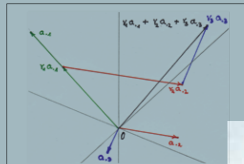
Bild 9: Eine geometrische Interpretation meiner "Kamm-Multiplikation" A \cdot v (3 Dimensionen)
