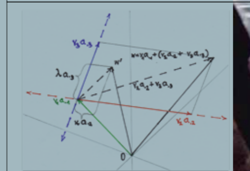
Bild 10: a' = \xi a_1 + \kappa a_2 + \lambda a_3 Ebene, die nicht durch den Ursprung geht
